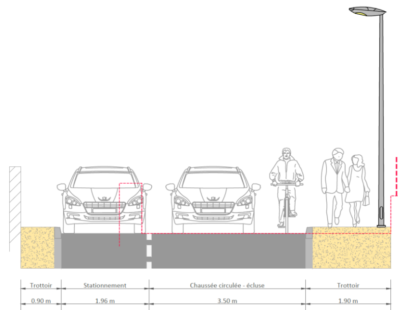
COUPE 5
