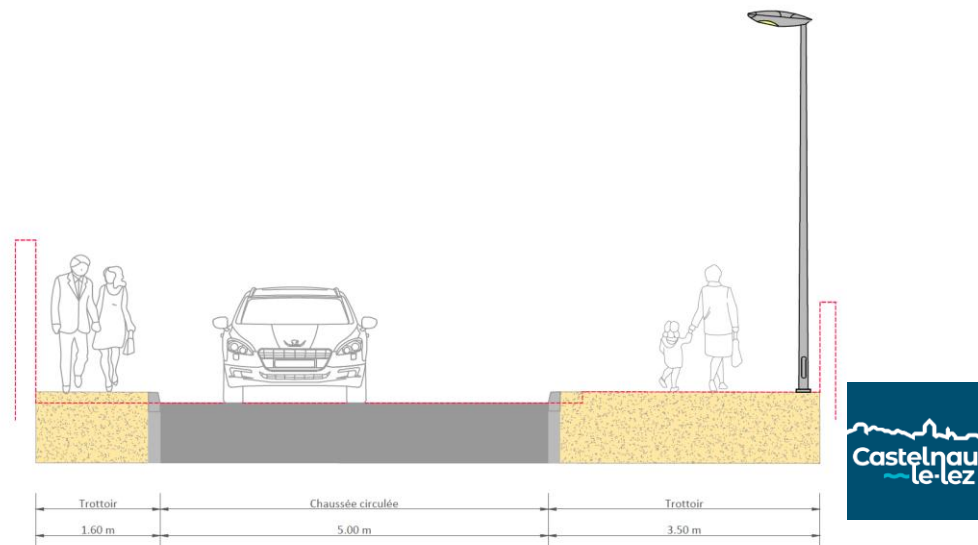
COUPE 7
