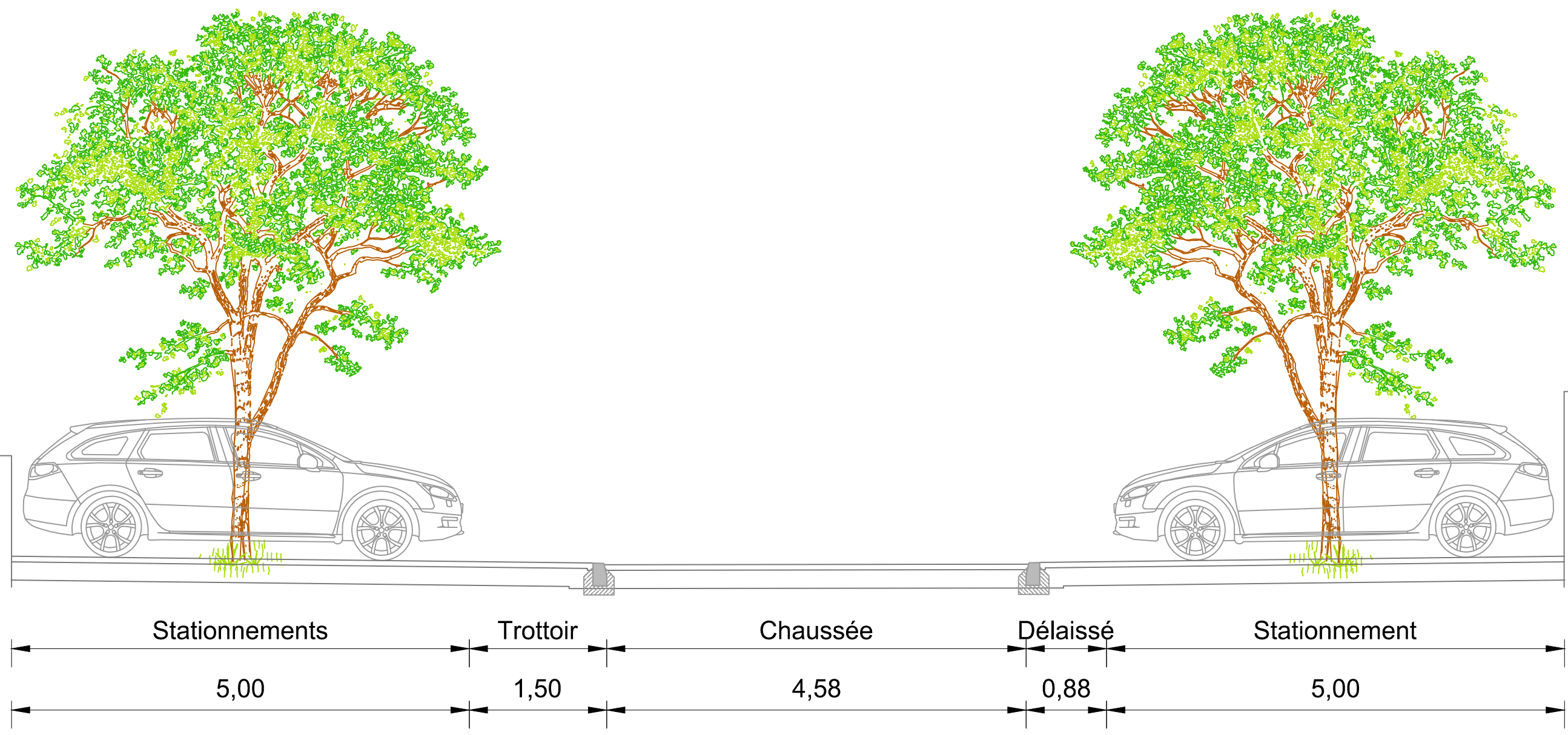
COUPE A-A : Trottoir ECHELLE : 1/50
